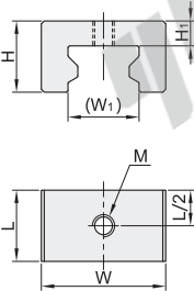
无防撞橡胶 ICG21
