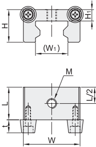
防撞橡胶头 ICG22
