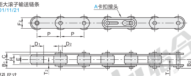
双节距大滚子全扣接头 VMV16
