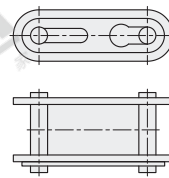
双节距大滚子全扣接头 VMV16
