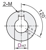
安装方式 (键槽+螺孔) N
