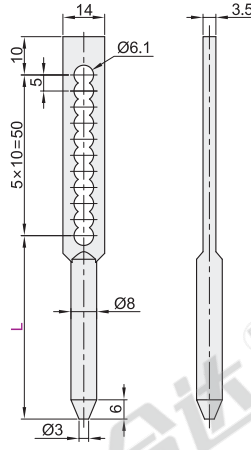
带多孔连杆 XAV51/XAV52
