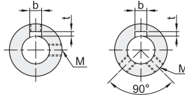
带*孔径的止动螺钉位于此处。
