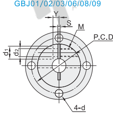
圆法兰型
