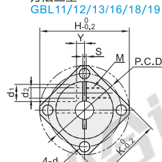
方法法兰型
