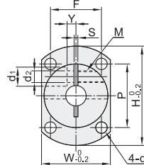
对边法兰型
