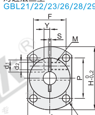
对边法兰型
