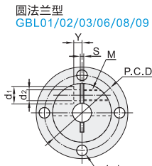
圆法兰型
