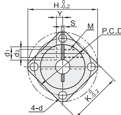
方法法兰型
