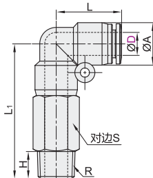
加长弯接头 XZS07
