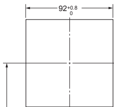
单独安装
