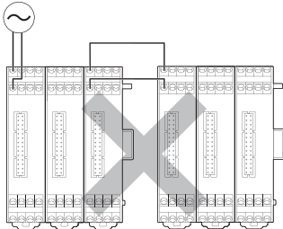
不正确
