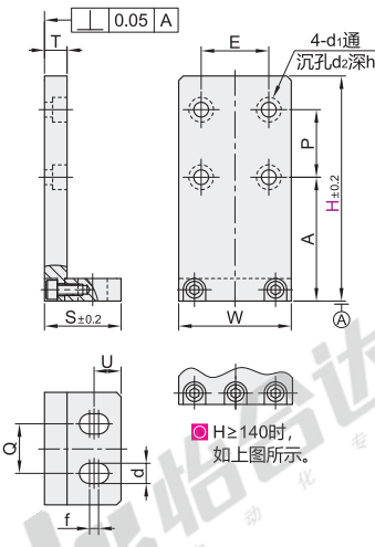
沉孔型 ZFG13/14/15/16
