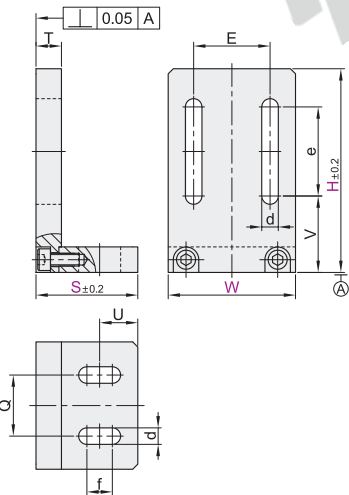
腰孔型 ZFG11/12
