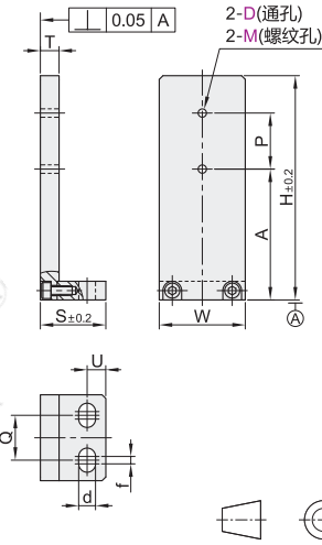
孔型选择型 ZFG17/18/19/20
