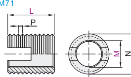
自攻开槽型
