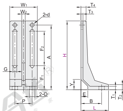
双腰孔型 WAQ12 WAQ22
