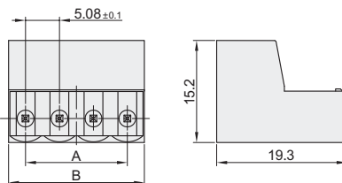
插座 ZKY14
