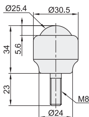
螺栓型 QDA13
