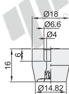
外径D: 14.82
