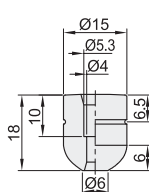
外径D: 15
