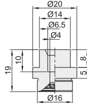
外径D: 16
