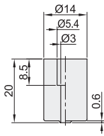
外径D: 14
