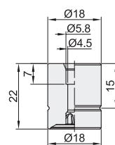
外径D: 18
