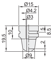
外径D: 9
