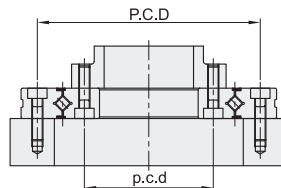
安装图
