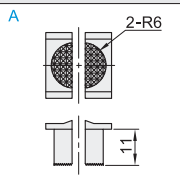
针轴前端形状
