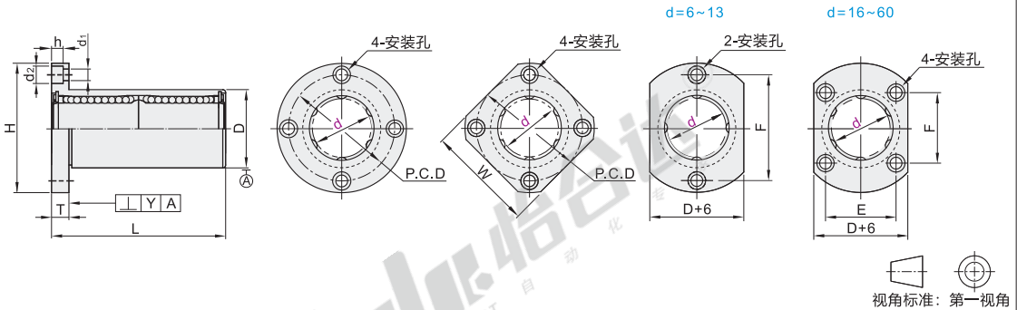
圆法兰型
