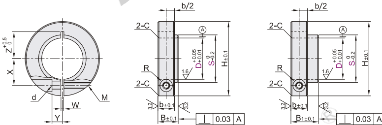
短压环型 FBH01/02/06
