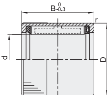
钢制簧片·带滚花 HF...-R
