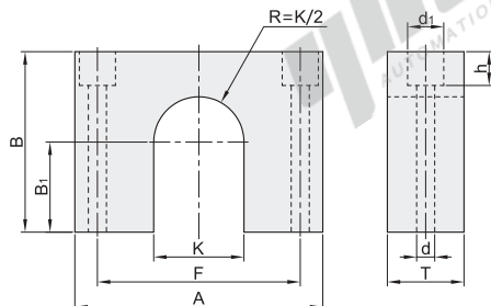
标准型 NDR51
