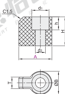
圆型 NDJ02
