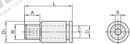
内六角孔直接头 XZH11
