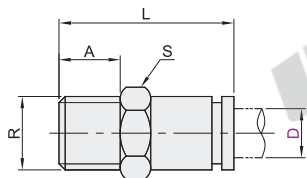
直接头 XZH01
