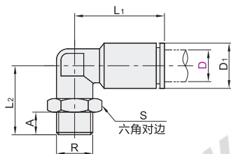
弯接头 XZH21
