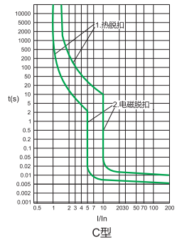
脱扣曲线图
