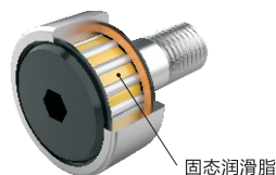
内部结构图
