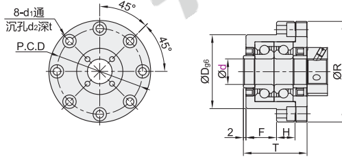
轴承组合形式: DF
