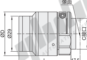
外形图：B
