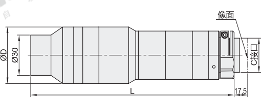
外形图：C
