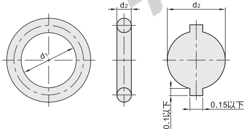
■ P系列O型圈 (JIS B 2401)
