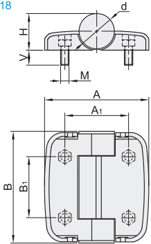
螺钉隐藏安装型 HFC18
