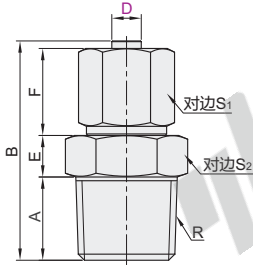
直接头 J-XYS01
