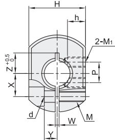
开口型-紧定螺钉锁紧型 FBA11/12/16
