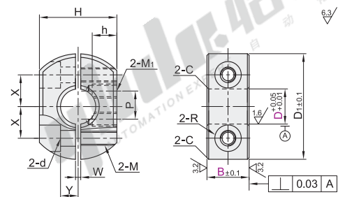
分离型-紧定螺钉锁紧型 FBA61/62/66
