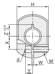
分离型-紧定螺钉锁紧型 FBA61/62/66
