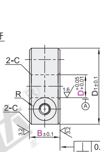
开口型-侧安装型 FBA21/22/26
