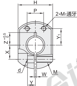
开口型-侧安装型 FBA21/22/26
