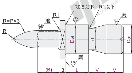
无肩型
