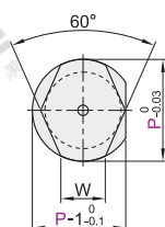
多棱型 YKD31/32/33
