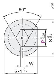
多棱型 YKD31/32/33
