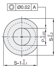
圆型 YKD01/02/03
