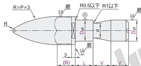
无肩型
