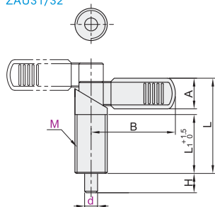
无锁紧螺帽 ZAU31/32
