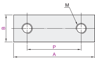
双螺孔型 TBL21/22/26
