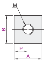
单螺孔型 TBL01/02/06
