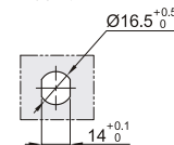
开孔尺寸
