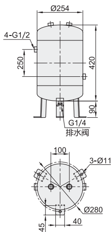
容积：20L
