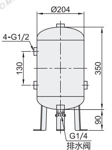
容积：10L
