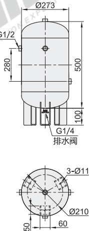
容积：30L
