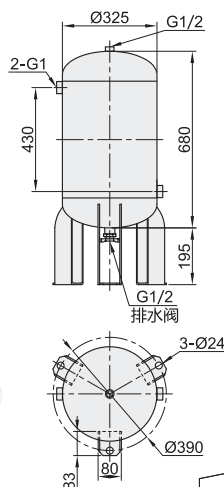
容积：55L
