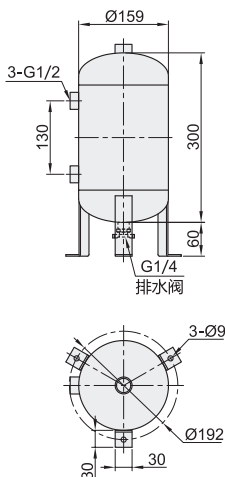
容积：5L
