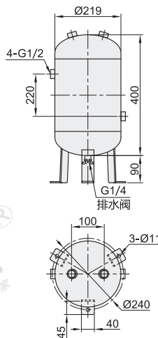
容积：15L
