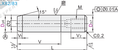
通孔螺纹型 BLX82/83
