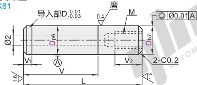
通孔螺纹型 BLX81
