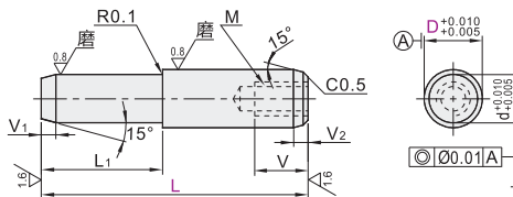
一端内螺纹型 BLY21/22/23
