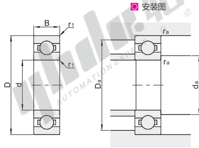
安装图
