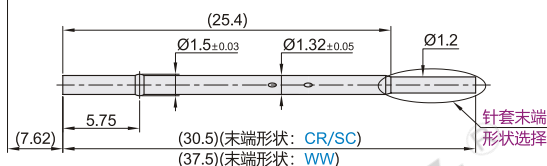
针套末端形状
