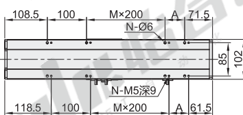
A向视图
