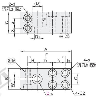
偏置型 RCG21/22
