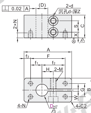
螺孔型 RCG11/12
