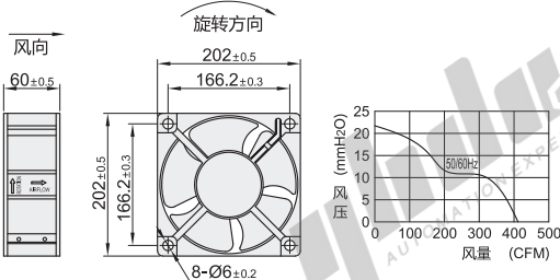
外形尺寸: 200
