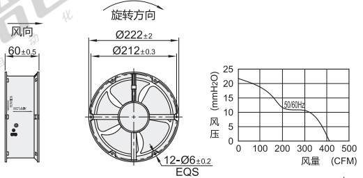
外形尺寸: 220
