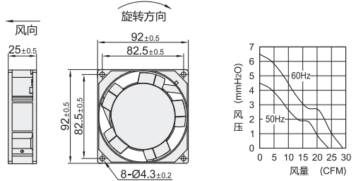
外形尺寸: 92
