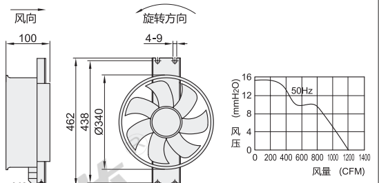
外形尺寸: 340
