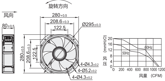
外形尺寸: 280
