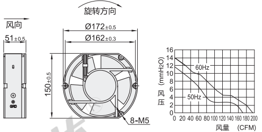
外形尺寸: 172
