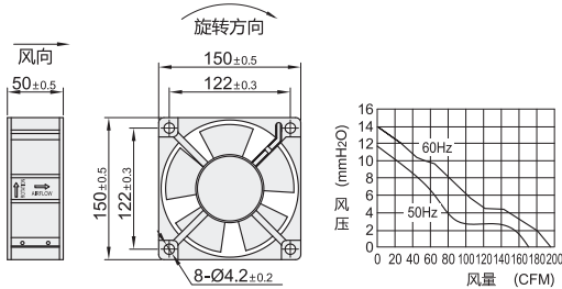
外形尺寸: 150
