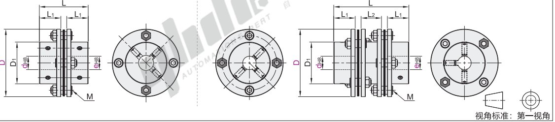
单膜片 DBN51
