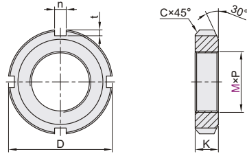
圆螺母 TBK74 TBK75
