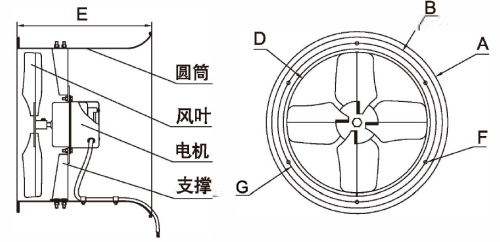
TA系列外形尺寸图
