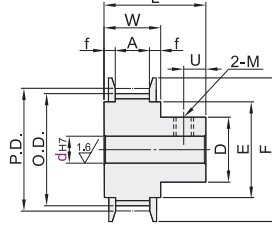
带轮形状：B形
