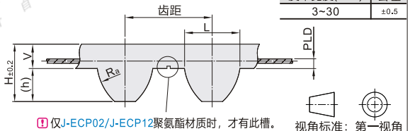
经济型 ECP01-S2M (齿距: 2)
