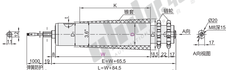
锥套尺寸表
