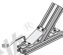
组装图
