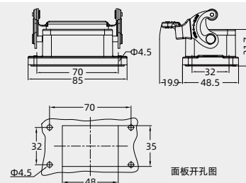
面板开孔图
