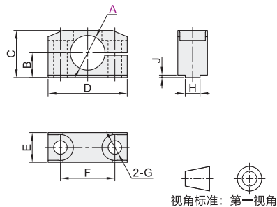
圆孔型 BWA10
