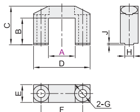
方槽型 BWA09
