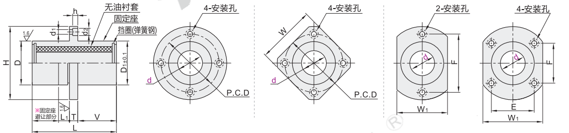
圆法兰型 E-OGJ01/02
