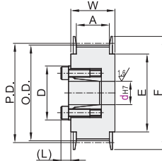
带轮形状
